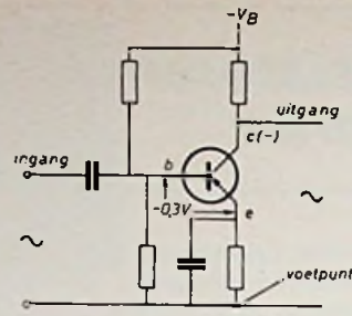
Fig. 1. Gemeenschappelijke emitterschakelingen met PNP transistoren.
